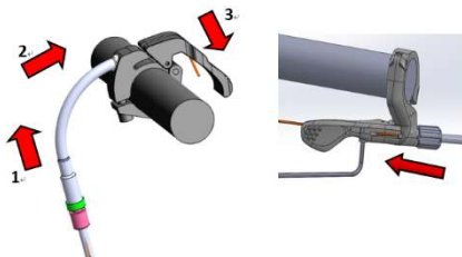
5-2 ケーブル ルート
